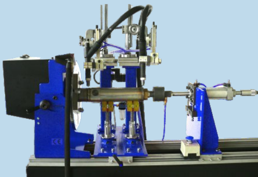
Механическая сварка круговыми швами
